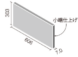
606×303 角片面小端仕上げ(右)
