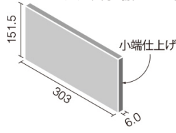
303×151 角片面小端仕上げ(短辺)
