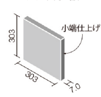
303 角片面小端仕上げ(右)
